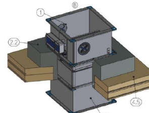
3D5.6.3. ábra. Tűzgátló csappantyú beépítése vasbeton gallerba CLT földem síkjára
