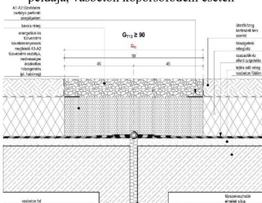
3F7 sz. ábra: extenzív zöldtető tetősíkból kiemelkedő tetőszinti tűzterjedés elleni gátja kialakításának példája
