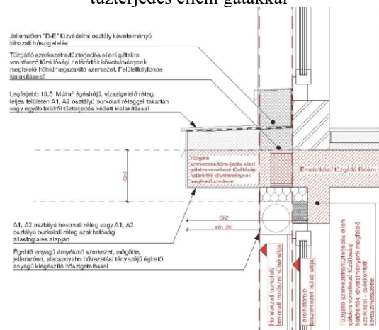
4F16 sz. ábra. Homlokzati tűzterjedés elleni gát geometriai értelmezése hőhidmegszakítóval és „D”-„E” tűzvédelmi osztályú lábazati hőszigeteléssel ellátott előtető vagy párkány esetén
