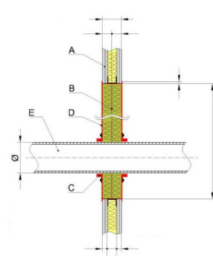
D1.1.1.4. ábra tűzgátló mandzsetta szerelt falban a lágy lezárás mindkét oldalára csavarozva
