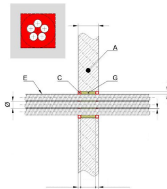
D1.1.3.2. ábra tűzvédelmi kiték lágy lezárásban (falárvezetés)
