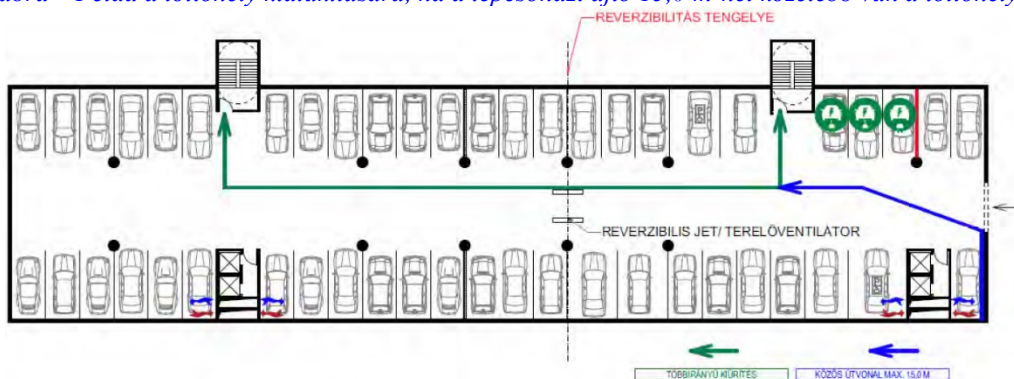
9. ábra Példa a többirányú kiürítés biztosítására
