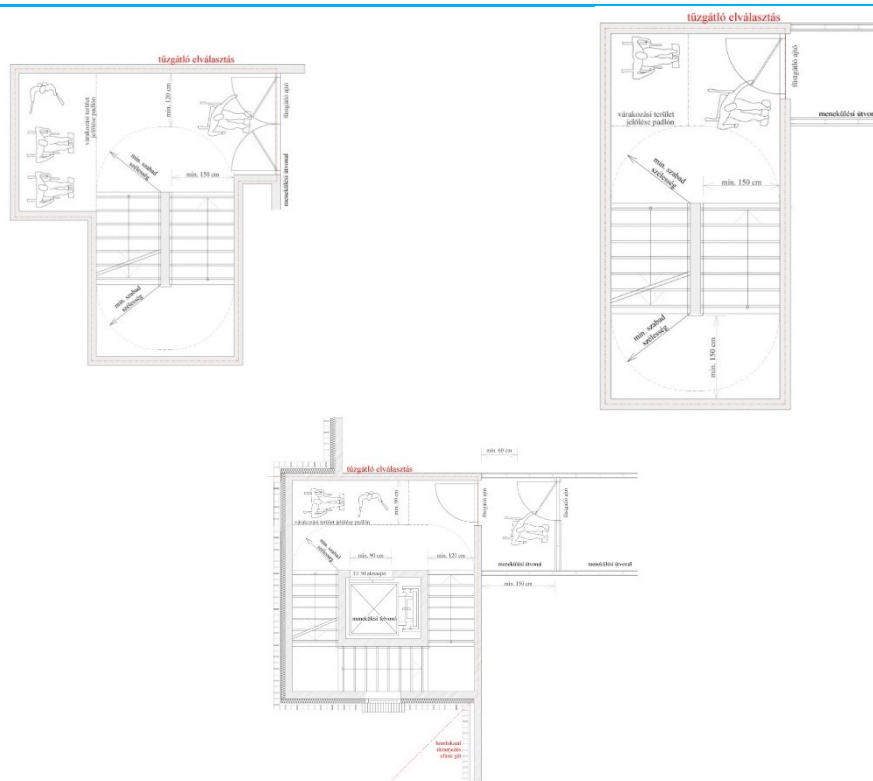
F4. ábra: A lépcsőház pihenőjének, illetve előterének átmeneti védett térként történő javasolt kialakítási lehetőségei
