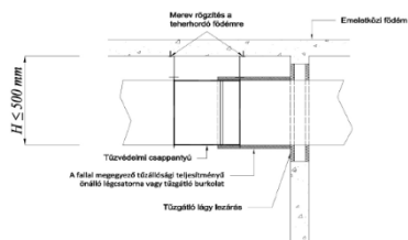
D5.5.1. ábra kis méretű csappantyú beépítése merev rögzítéssel tűzszakaszhatáron kívül
