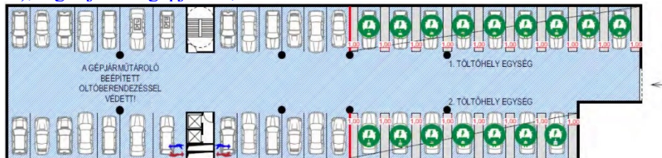
12. ábra – Példa a töltőhelyek kialakítására az a) pontban rögzített feltételek teljesülése esetén és a töltési pontonkénti teljesítmény nem haladja meg a 22 kW-ot
