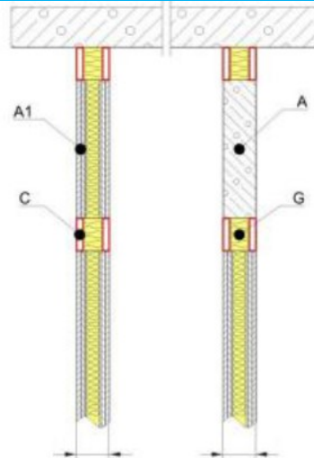
E3.2.4. ábra tűzvédelmi kitt (falban)
