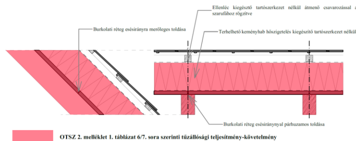
O5. sz. ábra: Látszó szarufás, kizárólag éghető anyagú hőszigeteléssel felépített, valós léptékű tüzteszttel minősített beépített tetőtéri rétegrend tűzállósági teljesítmény-követelményének értelmezése
