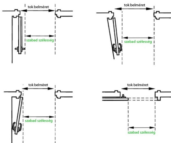
C8. ábra: 3Ajtók szabad szélessége meghatározásának elvei
