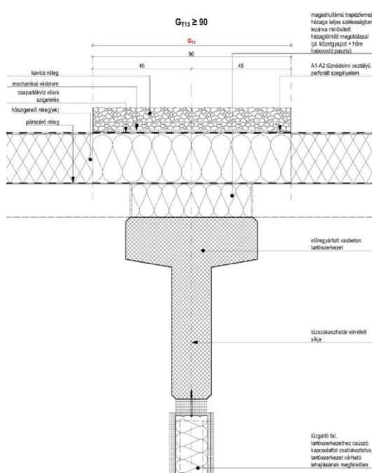
3F8 sz. ábra: előregyártott vasbeton vázszerkezetű és könnyű tetőfedém térelhatároló szerkezetű épület
