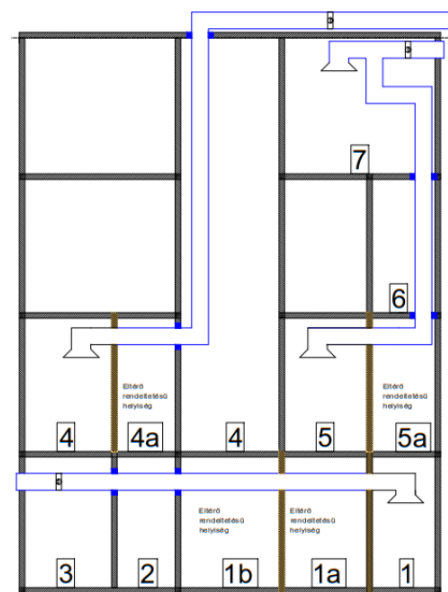
1 Tűzszakasz száma 2 Nagykonyhai elszívó ventilátor 3 Tűzgátló alapszerkezet MSZ EN 1366-1:2014+A1:2020 szerint éghető belső bevonattal vizsgált légszűrő, vagy légszűrő burkolat A mindeltett légszűrővel együttesen vizsgált tűzgátló reakciózó rendszer 1000°C feletti olvadáspontú, nem éghető anyagi légszűrő
