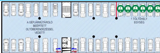
18. ábra – Példa a töltőhelyek kialakítására a c) pontban rögzített feltételek teljesülése esetén és a töltési pontonkénti teljesítmény nem haladja meg a 22 kW-ot
