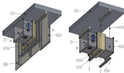
3D5.6.5. ábra. Tűzgátló csappantyú beépítése csúszó földépkapcsolattal és csappantyúbeépítő készlettel
