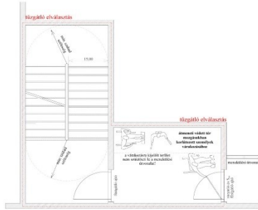
F3. ábra Független tűzszakasz-határral szintenként két tűzszakaszra osztott épületrész, két átmeneti védett tér és lépcsőház együttesével, mindkét oldalon menekülési felvonóval F4 A lépcsőház pihenőjének, illetve előterének átmeneti védett térként történő kialakítási lehetőségei
