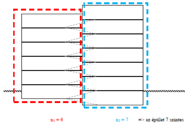
2. ábra: 1Példa felszinteltolásos épület szintszámának megállapítására
