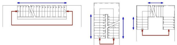
2 A ábra: 2 Lépcsőkarok és lépcsőkarok közötti útvonal hosszak
