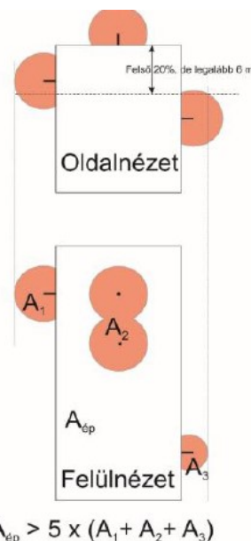
16. ábra: Vetületek figyelembe vétele
