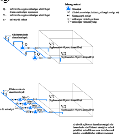
5. ábra: 3,4Példák a vízforrás kialakítására
