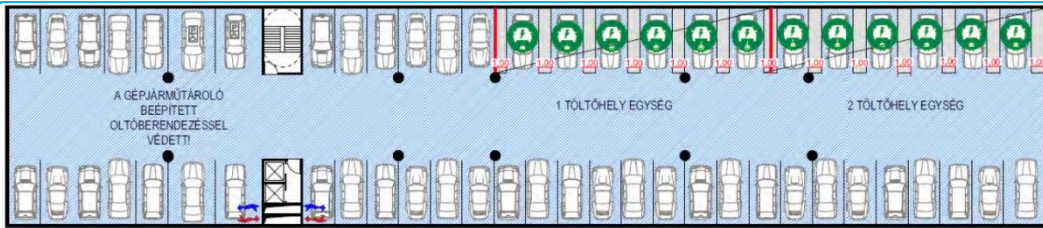
14. ábra – Példa a töltőhelyek kialakítására a közösségi rendeltetésű épületek gépjárműtárolói esetében, ahol a töltési pontonkénti teljesítmény meghaladja a 22 kW-ot, de legfeljebb 50 kW (DC) és az a) pontban rögzített feltételek teljesülésnek
