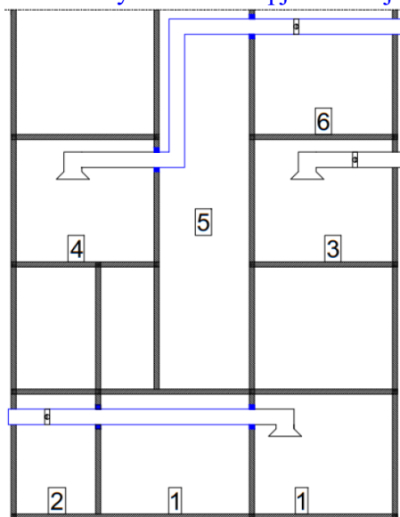
1 Tűzszakasz száma 2 Nagykonyhai elszívó ventilátor 3 Tűzgátló alapszerkezet MSZ EN 1366-1:2014+A1:2020 szerint éghető belső bevonattal vizsgált légszűrő, vagy légszűrő burkolat A mindeltett légszűrővel együttesen vizsgált tűzgátló reakciózó rendszer 1000°C feletti olvadáspontú, nem éghető anyagi légszűrő
