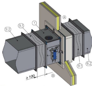
1: tűzgátló csappantyú 9.1: hőtágulási kompenzátorok 9.2: acél szellőző légszatórna A: beépítés oldál B: kezelő oldal
