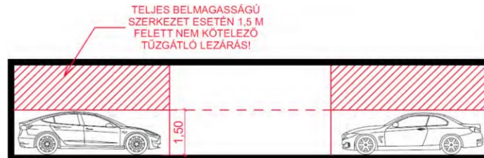
23. ábra – Teljes belmagasságú fix leválasztásra vonatkozó feltétel
