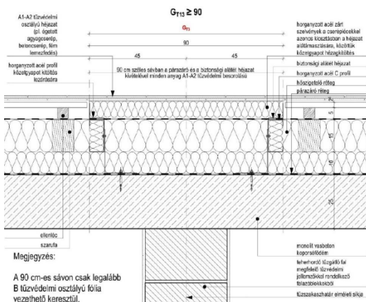
3F5 sz. ábra: magastető tetősíkból kiemelkedő tetőszinti tűzterjedés elleni gátja kialakításának példája, vasbeton koporsófedém esetén
