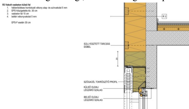
E6 sz. ábra. Falazott, vakolt homlokzati hőszigetelő rendszerrel ellátott fal ablakcsatlakozása társított árnyékoló szerkezettel
