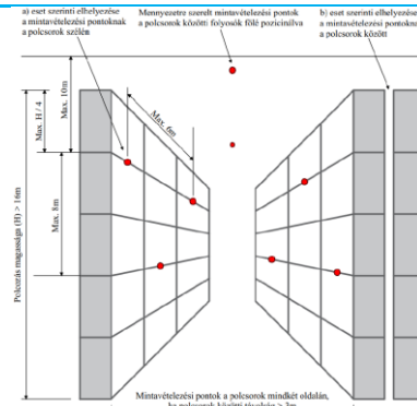
9. ábra: Polcközi védelem kialakítása
