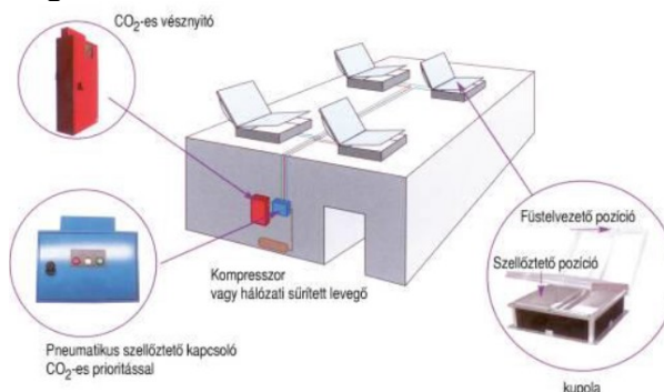
1.32b. ábra: Példa munkahengeres vésznyitás és munkahengeres szellőztetés megoldására
