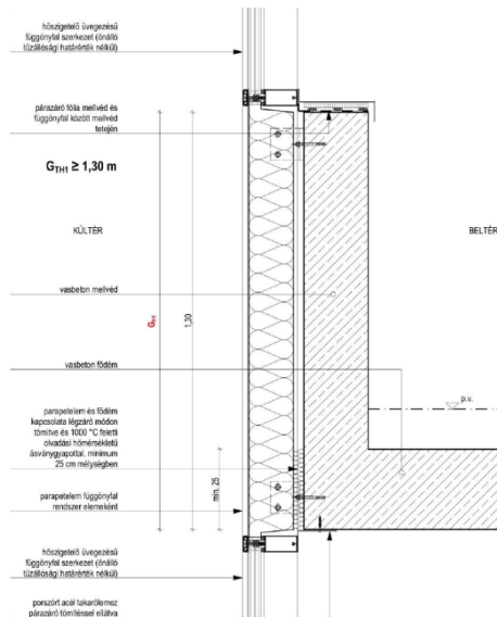
3F11 sz. ábra: tűzállósági teljesítmény nélküli függőfalról független, a tűzgátló födémmel folytonos egységet alkotó, önálló tűzállósági teljesítményű parapetfal, mint homlokzati tűzterjedés elleni gát példája
