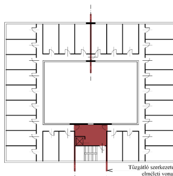
F2.5. ábra Független tűzszakasz-határral szintenként két tűzszakaszra osztott, körbejárható, nyitott belső udvart tartalmazó épület egy átmeneti védett tér és lépcsőház együttesével
