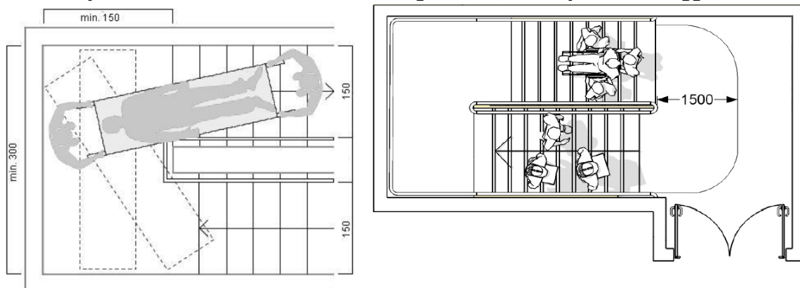
5A. ábra: Kerekesszékekkel és hordágygal történő mentésre alkalmas lépcsőház minimális méretei
