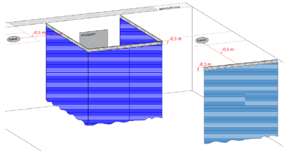
5B. ábra: Pontszerű érzékelő elhelyezése térelválasztó elem (függöny) esetén
