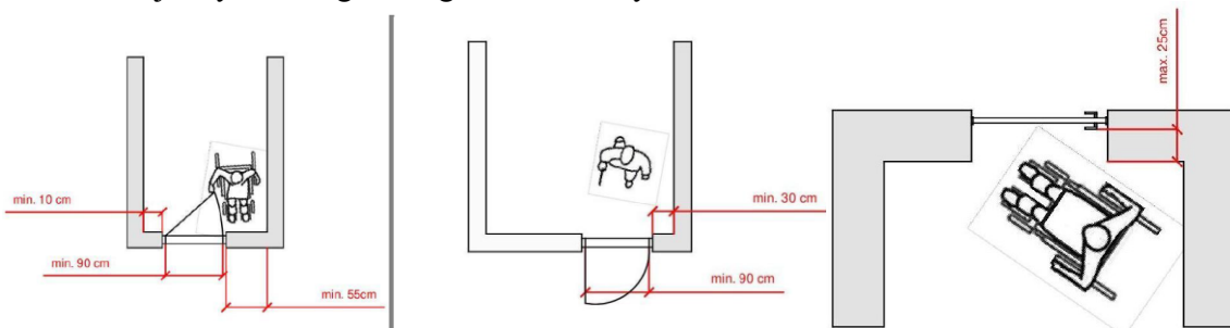
6A. ábra: Példák az akadálymentesen használható ajtók megközelítési útvonalának kialakítására
