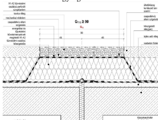
3F6 sz. ábra: extenzív zöldtető tetősíkból kiemelkedő tetőszinti tűzterjedés elleni gátja kialakításának példája
