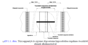
2D5.1.1. ábra. Tűzcsappantyú és egyenes légszatórna kapcsolódása rugalmas összekötő elem alkalmazásával
