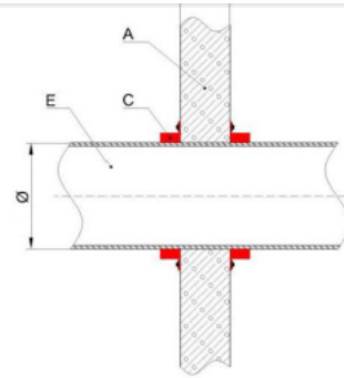
D1.1.1.2. ábra tűzgátló mandzsetta épített fal mindkét oldalára csavarozva
