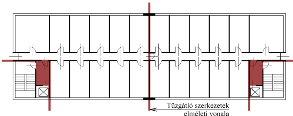
F3. ábra Független tűzszakasz-határral szintenként két tűzszakaszra osztott épületrész, két átmeneti védett tér és lépcsőház együttesével, mindkét oldalon menekülési felvonóval F4 A lépcsőház pihenőjének, illetve előterének átmeneti védett térként történő kialakítási lehetőségei
