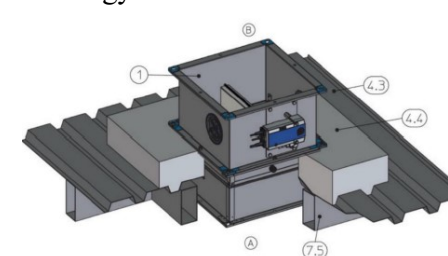
3D5.6.4. ábra. Tűzgátló csappantyú beépítése vasbeton gallerba könnyűszerkezetes földem síkjára
