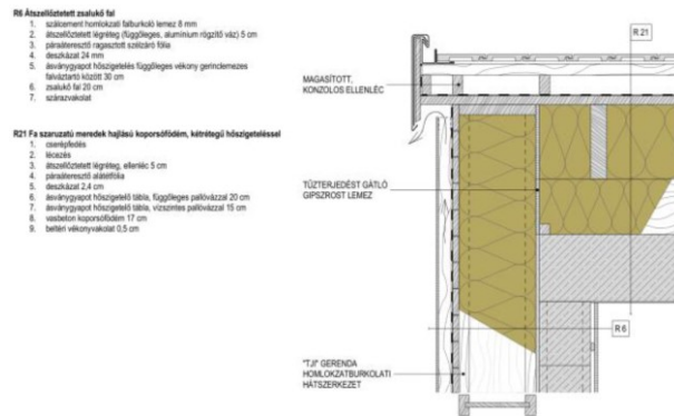
E3 sz. ábra. Falazott, átszellőztetett légréses homlokzatburkolattal ellátott fal és átszellőztetett légréses magasetető csatlakozása
