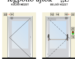
G21. ábra: Egyszárnyú, elektromos zárással rendelkező homlokzati ajtók / tűzgátló vagy lépgömb ajtók – „E” típus
