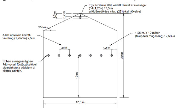
1a. ábra: 2Vonali füstérzékelő elhelyezése dőlt födém vagy mennyezet esetén
