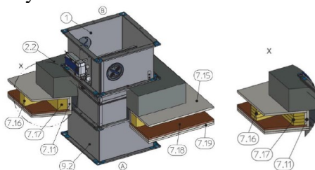
3D5.6.2. ábra. Tűzgátló csappantyú beépítése vasbeton gallerba egy fagerendás földem síkjára
