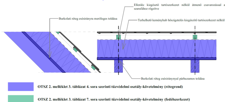
O6. sz. ábra: Látszó szarufás, kizárólag éghető anyagú hőszigeteléssel felépített, valós léptékű tüzteszttel minősített beépített tetőtéri rétegrend tűzvédelmi osztály-követelményének értelmezése
