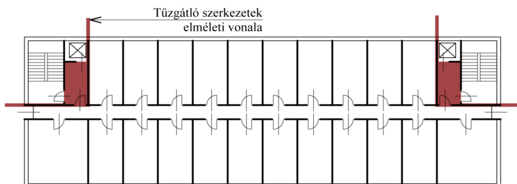
F2.2. ábra Függőleges tűzszakasz-határral szintenként két tűzszakaszra osztott épület egy átmeneti védett tér és lépcsőház együttesével
