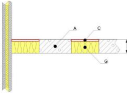
E3.2.3. ábra tűzvédelmi kitt (födém)
