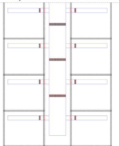
J-1 ábra (metszet) E600 x S single légszatórna (MSZ EN 1366-9, MSZ EN 13501-4)
