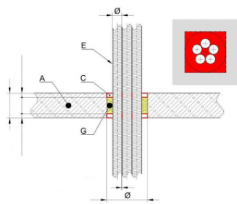
D1.1.3.1. ábra tűzvédelmi kiték lágy lezárásban (födémárvezetés)
