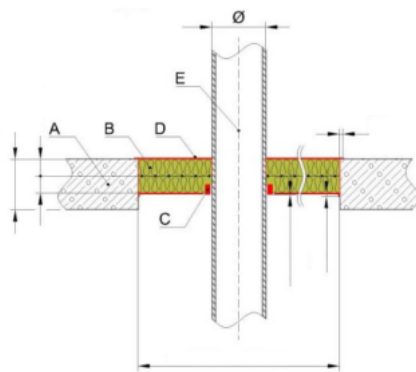
D1.1.1.3. ábra tűzgátló mandzsetta lágy lezárásban a földem síkján belül
