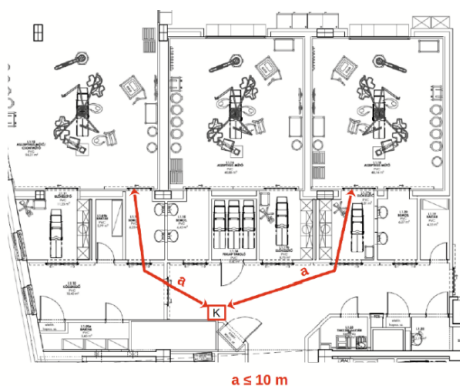
9. ábra – Kézi jelzésadó elhelyezése a műtő helyiségcsoportnál
