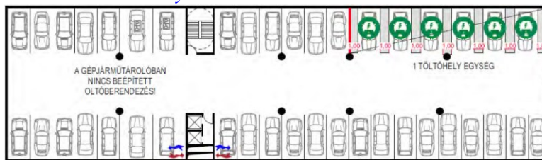
16. ábra – Példa a töltőhelyek kialakítására a b) pontban rögzített feltételek teljesülése esetén és a töltési pontonkénti teljesítmény nem haladja meg a 22 kW-ot
