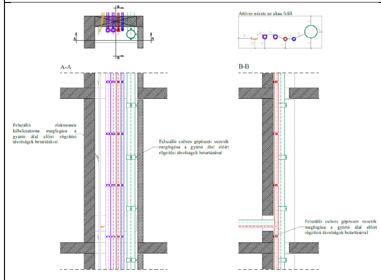
L/I.2. ábra - Gépészeti és villamos szerelés készen, tűzvédelmi lezárások elhelyezése előtti állapot
