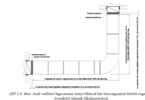
2D5.1.6. ábra. Acél szellőző légszatórna irányváltással két tűzcsappantyú között rugalmas összekötő elem alkalmazásával
