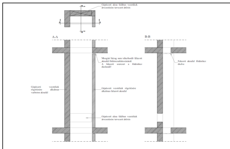
L/I.1. ábra - Szerelőakna szerkezetkész állapotban, a gépészeti és villamos szerelés megkezdése előtt
