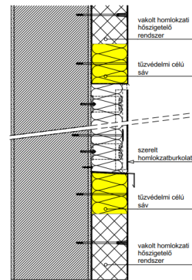
4.3.3.16. 2. és 3. ábra 4 Vegyes kialakítású homlokzati felületek elválasztásának vízszintes és függőleges részletrajzai tűzvédelmi sávokkal
