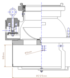
24. ábra szűrőkosár
