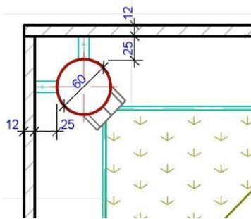
1. ábra: Kéménycsövek SBI vizsgálati mintájának lehetséges elrendezései
