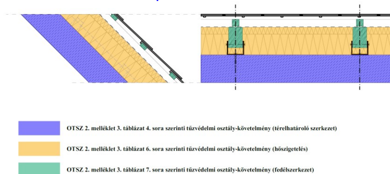
O12. sz. ábra: Vasbeton koporsófödém fölé épített ácsszerkezetű fedélszerkezettel és rétegrenddel képzett tetőfödém tűzvédelmi osztály- követelményének értelmezése beépített tetőtér esetén
