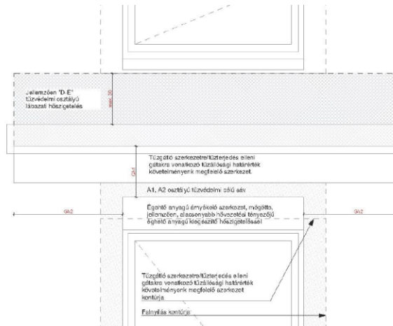
4F16 sz. ábra. Homlokzati tűzterjedés elleni gát geometriai értelmezése hőhíd megszakítóval és „D”-, „E” tűzvédelmi osztályú lábazati hőszigeteléssel ellátott előtető vagy párkány esetén
