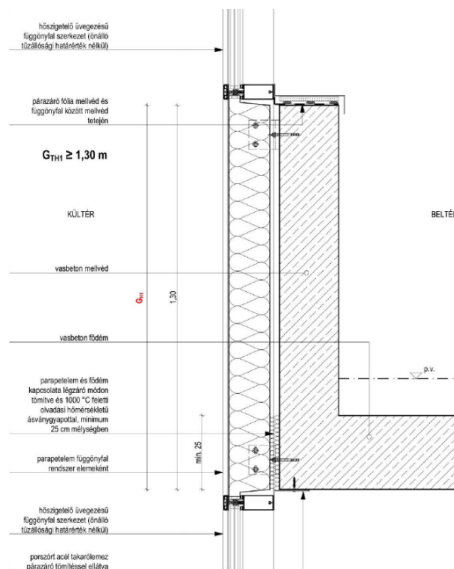
F11 sz. ábra: tűzállósági teljesítmény nélküli függőnyfaltól független, a tűzgátló földemmel folytonos egységet alkotó, önálló tűzállósági teljesítményű parapetfal, mint homlokzati tűzterjedés elleni gát példája
