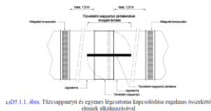
2D5.1.1. ábra. Tűzcsappantyú és egyenes légcsatorna kapcsolódás rugalmas összekötő elemek alkalmazásával
