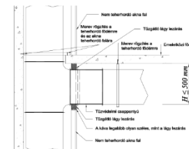
2D5.3.4. ábra. Nem teherhordó aknafalban épített kis méretű tűzvédelmi csappantyú a födémhez és az akna teherhordó falához mereven rögzített légszűrőkkel
