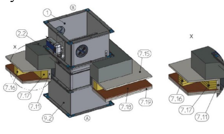
3D5.6.2. ábra. Tűzgátló csappantyú beépítése vasbeton gallerba egy fagerendás földem síkjára
