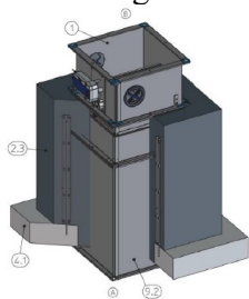
3D5.6.1. ábra. Tűzgátló csappantyú beépítése vasbeton gallerba a vasbeton földem síkjától távol
