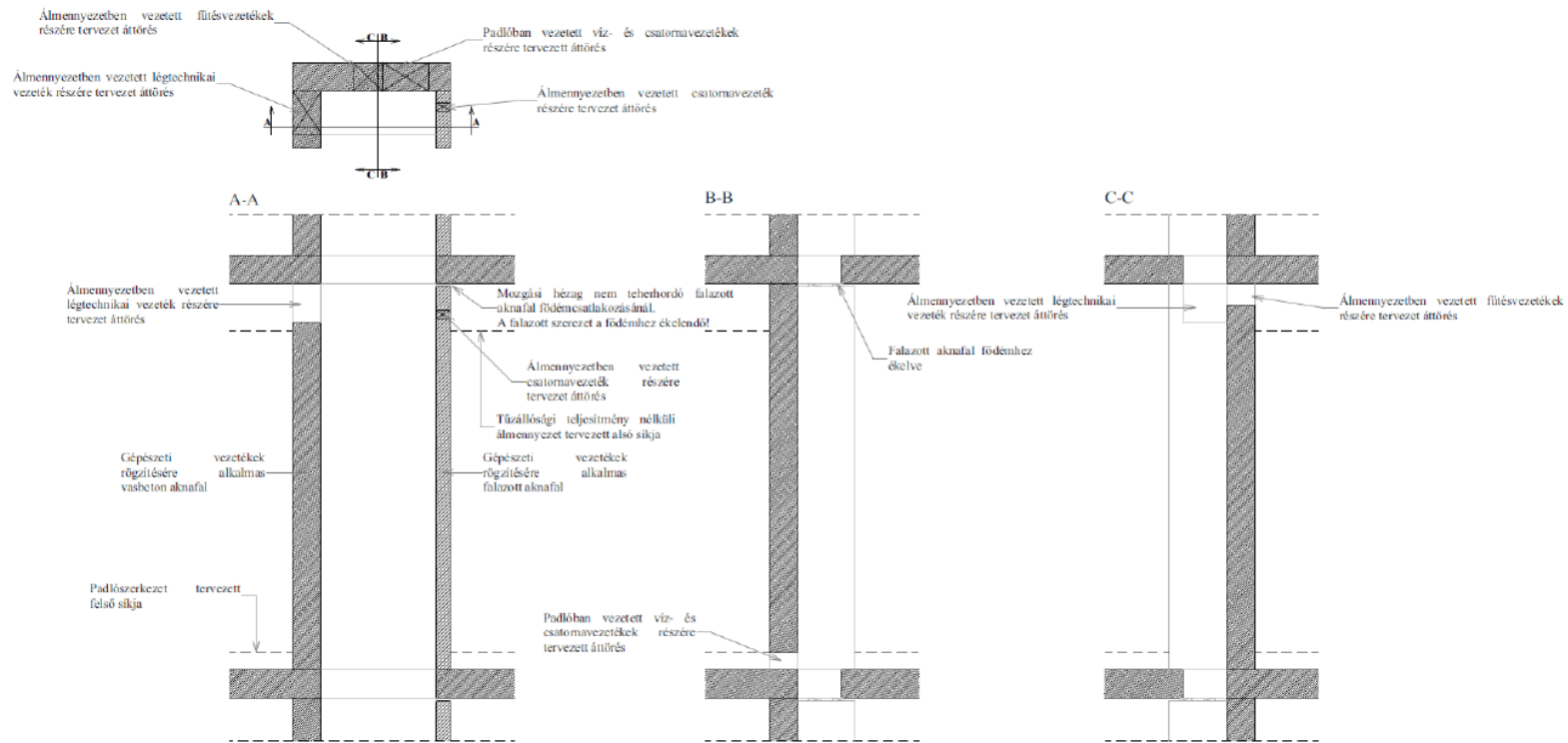
L/II.1. ábra - Szerelőakna szerkezetkész állapotban, a gépészeti és villamos szerelés megkezdése előtt
