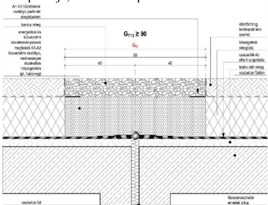
3F5 sz. ábra: magastető tetősíkbán tartott tetőszinti tűzterjedés elleni gátja kialakításának példája, vasbeton koporsófödém esetén
