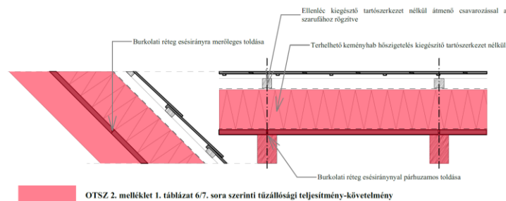
O5. sz. ábra: Látszó szarufás, kizárólag éghető anyagú hőszigeteléssel felépített, valós léptékű tűztesztel minősített beépített tetőtéri rétegrend tűzállósági teljesítmény-követelményének értelmezése
