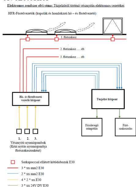
K.1.2-1 ábra: Automatikus (tűzjelző érzékelő általi) vésznyitás megoldásának példája
