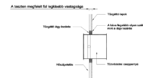
D5.4.2. ábra. Legalább 100 mm vastag szerelt falba épített csappantyú beépítése lágy lezárással
