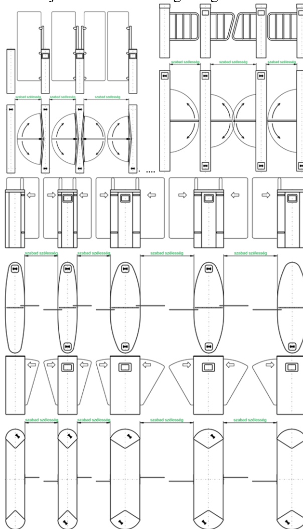
2C9 ábra: Beléptető kapuk szabad nyílászélességének megállapítása
