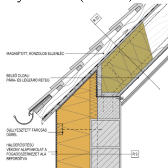
E2 sz. ábra. Falazott, éghető hőszigeteléssel ellátott fal és átszellőztetett légrése magastető csatlakozása
