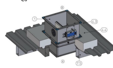
3D5.6.4. ábra. Tűzgátló csappantyú beépítése vasbeton gallerba könnyűszerkezetes földem síkjára
