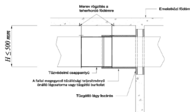
D5.5.1. ábra kis méretű csappantyú beépítése merev rögzítéssel tűzszakaszhatáron kívül
