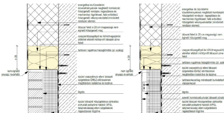
M3 ábra Csomópont javasolt elvi kialakítása légréses lábhatatok esetében
