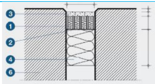
E3.3.1. ábra habosodó hézagtömítő elem
