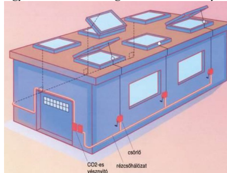
1,2,32a. ábra: Csörlő és CO 2 távnyitás megoldásának példája
