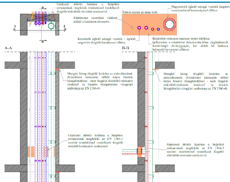
L/I.3. ábra - Tűzgátló lezárások készen, akna lezárása előtti állapot
