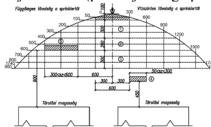
1. ábra ESFR fej szórásképi akadályok
