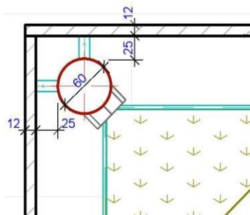
1. ábra: Kéménycsövek SBI vizsgálati mintájának lehetséges elrendezései
