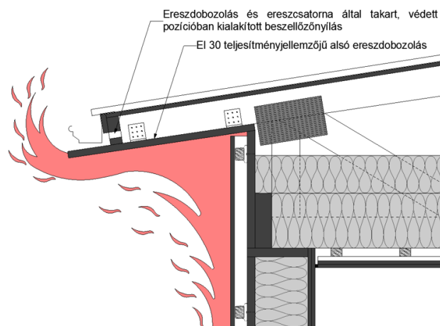
O14. sz. ábra: Homlokzat síkja elé lógó ereszt tűzvédelmileg megfelelő elvi kialakítása
