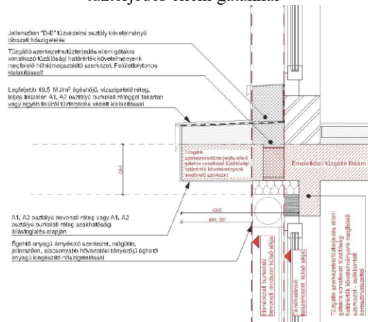
4F16 sz. ábra. Homlokzati tűzterjedés elleni gát geometriai értelmezése hőhíd megszakítóval és „D”-, „E” tűzvédelmi osztályú lábazati hőszigeteléssel ellátott előtető vagy párkány esetén
