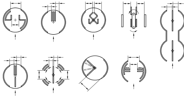
C10. ábra: 4Forgóajtók nyílás szélességének meghatározása
