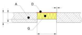
E3.1.3. ábra tűzvédelmi bevonat (földemben)
