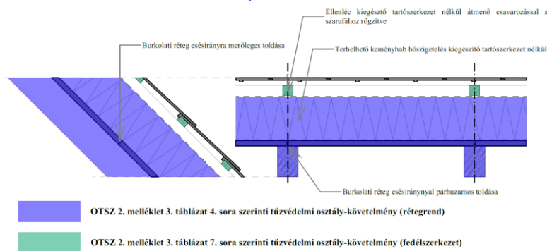
O6. sz. ábra: Látszó szarufás, kizárólag éghető anyagú hőszigeteléssel felépített, valós léptékű tűztesztel minősített beépített tetőtéri rétegrend tűzvédelmi osztály-követelményének értelmezése
