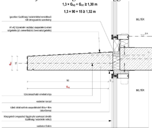
F9 sz. ábra: lapostetők vízvezetése és a tűzterjedés elleni gátak összefüggései
