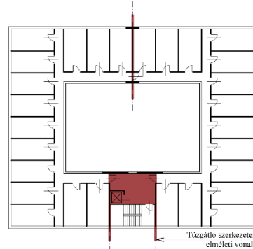
F2.5. ábra Függőleges tűzszakasz-határral szintenként két tűzszakaszra osztott, körbejárható, nyitott belső udvart tartalmazó épület egy átmeneti
