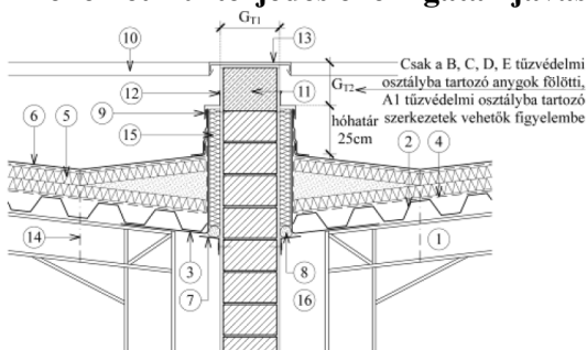
F1 sz. ábra: lapostető tetőszinti tűzterjedés elleni gátjának példája, egyszeres tűzfal
