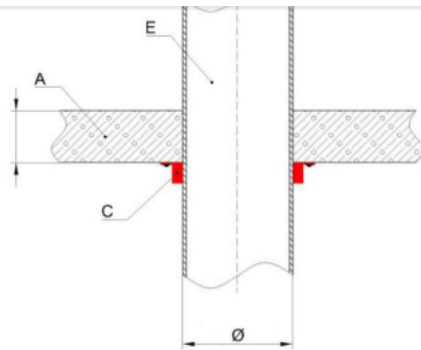
D1.1.1.1. ábra tűzgátló mandzsetta földem alá csavarozva
