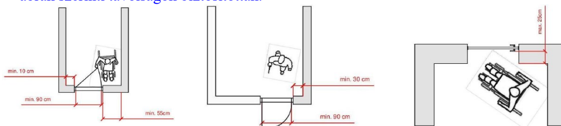
7A. ábra: 4Példák az akadálymentesen használható ajtók megközelítési útvonalának kialakítására
