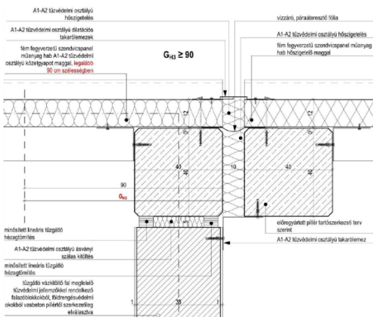
F12 sz. ábra: előregyártott vasbeton pillérvázás tartószerkezetéhez közetgyapot maghőszigetelésű szendvicspanelből kialakított homlokzati
