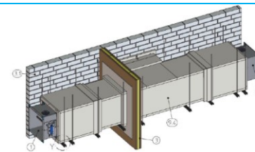
D5.5.3. ábra. Tűzgátló csappantyú beépítése külön függesztéssel a tűzszakaszhatár(ok) síkjától távol
