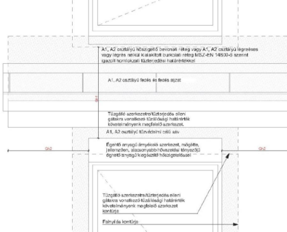
4F17 sz. ábra. Homlokzati tűzterjedés elleni gát geometriai értelmezése hőhíd megszakítóval és „D”-, „E” tűzvédelmi osztályú lábazati hőszigeteléssel ellátott előtető vagy párkány esetén
