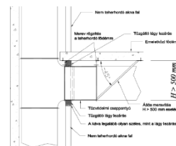
2D5.3.3. ábra. Nem teherhordó aknafalban épített, a födémhez mereven rögzített nagy méretű tűzvédelmi csappantyú
