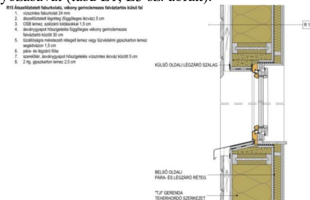
E4 sz. ábra. Szerelt, átszellőztetett légréses homlokzatburkolattal ellátott fal ablakesatlakozása
