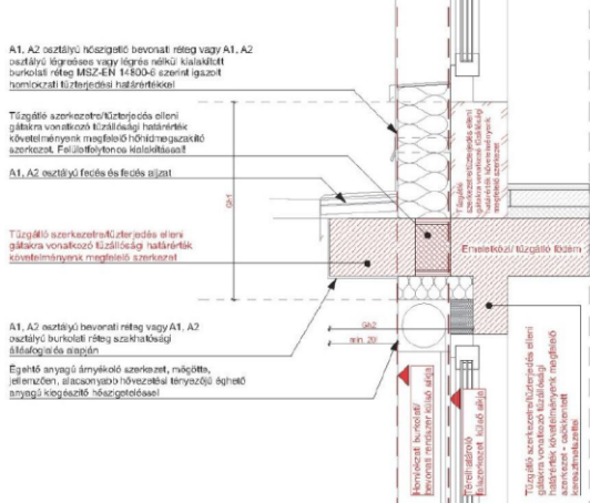
4F17 sz. ábra. Homlokzati tűzterjedés elleni gát geometriai értelmezése hőhíd megszakítóval és „D”-, „E” tűzvédelmi osztályú lábazati hőszigeteléssel ellátott előtető vagy párkány esetén
