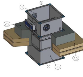
3D5.6.3. ábra. Tűzgátló csappantyú beépítése vasbeton gallerba CLT földem síkjára
