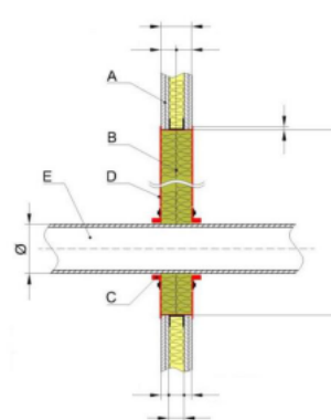
D1.1.1.4. ábra tűzgátló mandzsetta szerelt falban a lágylezárás mindkét oldalára csavarozva
