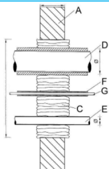
D3.5. ábra Vegyes tűzgátló lezárás (cső és kábel egy áttörésben) tűzvédő lezárása zsákokkal
