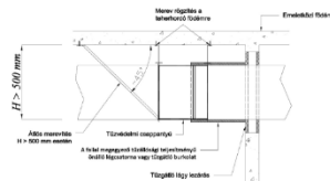
D5.5.2. ábra. Nagyméretű csappantyú beépítése merev rögzítéssel tűzszakaszhatáron kívül
