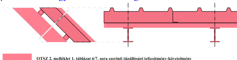
O1. sz. ábra: Fémfegyverzetű szendvicspanelből kialakított tetőfödém tűzvédelmi
