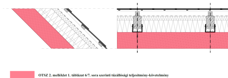
O11. sz. ábra: Vasbeton koporsófödém fölé épített ácsszerkezetű fedélszerkezettel és rétegrend-del képzett tetőfödém tűzállósági teljesítmény- követelményének értelmezése beépített tetőtér esetén
