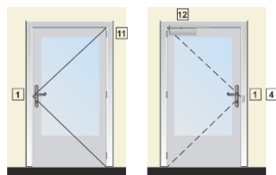
G1. ábra: Egyszárnyú, zárás nélküli belső ajtók / tűzgátló ajtók – „A” típus
