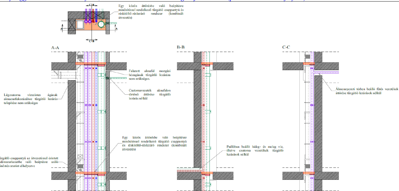
L/III.3. ábra - Tűzgátló lezárások készen, akna lezárása előtti állapot
