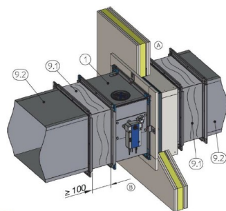
1: tűzgátló csappantyú 9.1: hőtágulási kompenzátorok 9.2: acél szellőző légcsatorna A: beépítési oldal B: brezelő oldal
