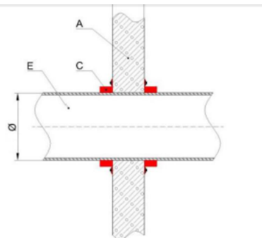
D1.1.1.2. ábra tűzgátló mandzsetta épített fal mindkét oldalára csavarozva
