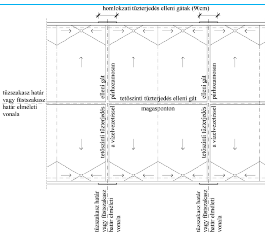
F9 sz. ábra: lapostetők vízvezetése és a tűzterjedés elleni gátak összefüggései
