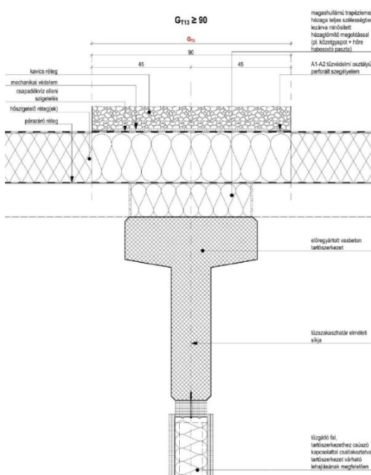
3F8 sz. ábra: előregyártott vasbeton vázszerkezetű és könnyű tetőfödém térelhatároló szerkezetű épület tűzszakaszhatárához kapcsolódó síkban tartott tetőszinti tűzterjedés elleni gátjának példája
