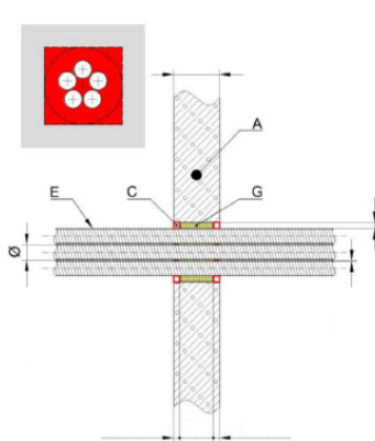
D1.1.3.2. ábra tűzvédelmi kiték lágy lezárásban (falátvezetés)
