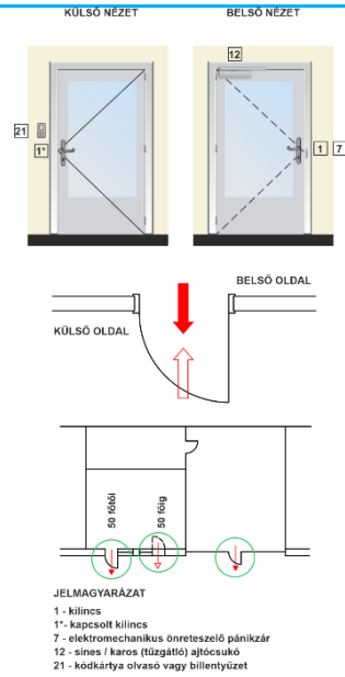
G18. ábra: Egyszárnyú, elektromos zárassal rendelkező homlokzati ajtók / tűzgátló ajtók – „B” típus
