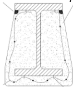
H2. sz. ábra: dobozos profiltényező használata habarcsvédelem esetén
