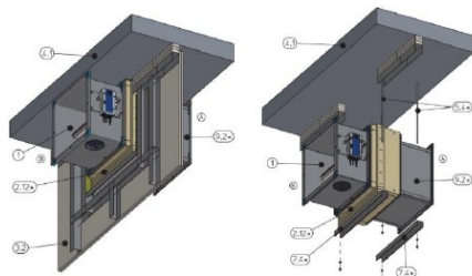
3D5.6.5. ábra. Tűzgátló csappantyú beépítése csúszó földépcsővel és csappantyúbeépítő készlettel
