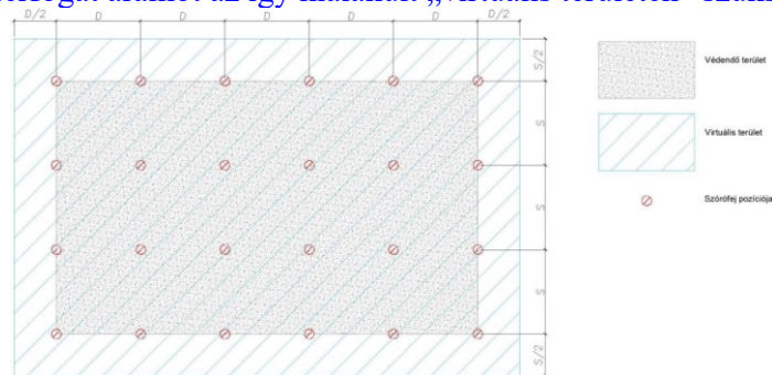
4. ábra: 3Nyitott szórófejes habbaloltó berendezés szórófej kiosztás
