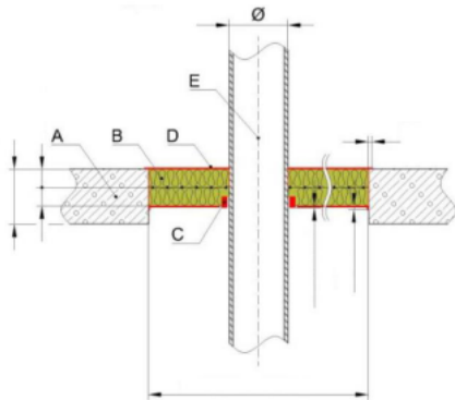
D1.1.1.3. ábra tűzgátló mandzsetta lágylezárásban a földem síkján belül
