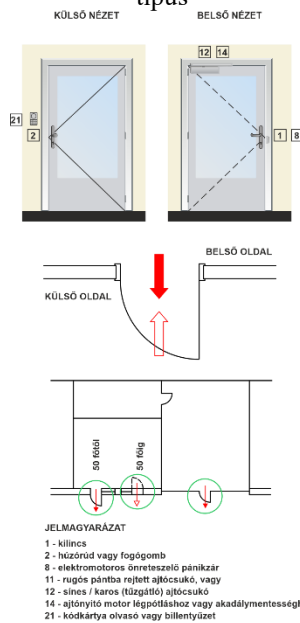
G19. ábra: Egyszárnyú, elektromos zárassal rendelkező homlokzati ajtók / légpótló ajtók – „C” típus
