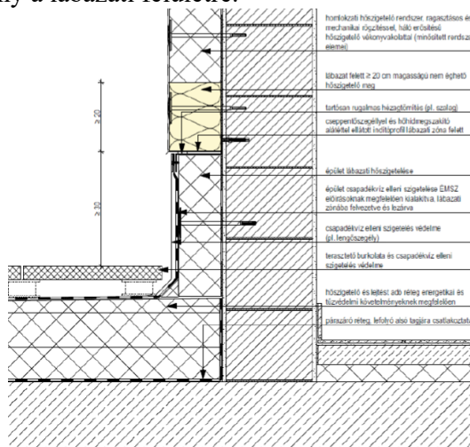
M2 ábra Terasztető lábhatati csomópontjának elvi kialakítása
