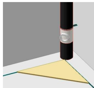
1. ábra: Kéménycsövek SBI vizsgálati mintájának lehetséges elrendezései
