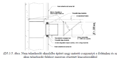
D5.3.5. ábra. Nem teherhordó aknafalba épített nagy méretű csappantyú a földéhez és az akna teherhordó falához mereven rögzített légesatornákkal
