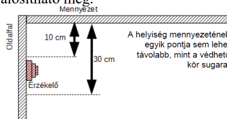
8. ábra Érzékelő oldalfalra szerelése
