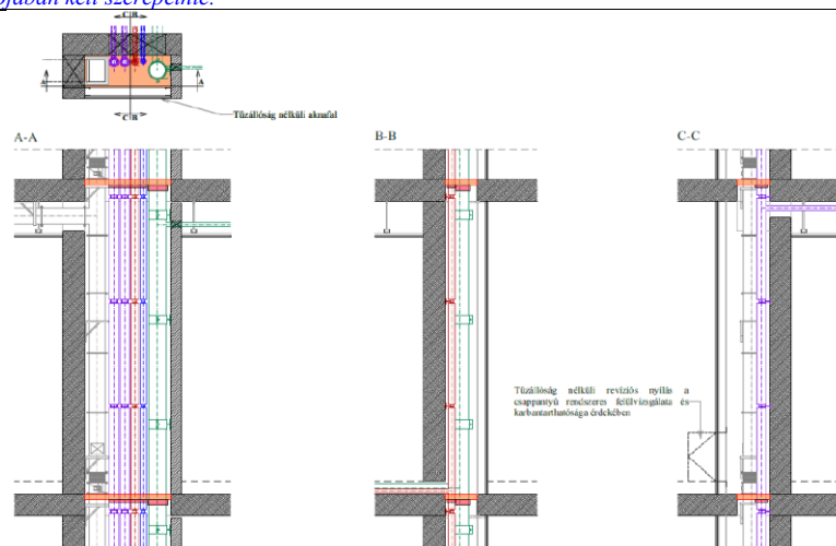
L/III.4. ábra - Szerelés érdekében nyitva hagyott aknafal lezárva, akna készre kivitelezve
