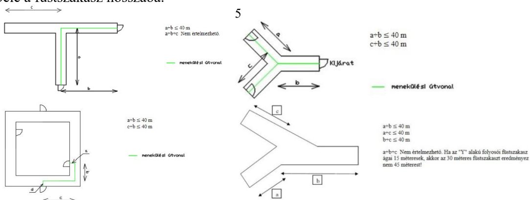
13-6. ábra: folyosói füstszakasz hosszúsága
