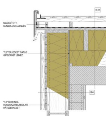
E3 sz. ábra. Falazott, átszellőztetett légréses homlokzatburkolattal ellátott fal és átszellőztetett légréses magastető csatlakozása
