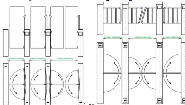
C8. ábra: 3Ajtók szabad szélessége meghatározásának elvei
