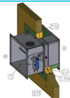
3D5.6.7. ábra. Tűzgátló csappantyú száraz (lágylezárásos) beépítése CLT fal síkján belül
