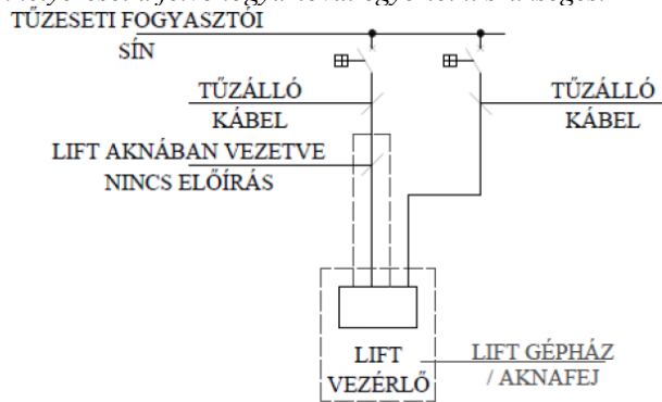
(A) LIFT VEZÉRLŐBEN AZ ÁTKAPCSOLÓ 10. ábra
