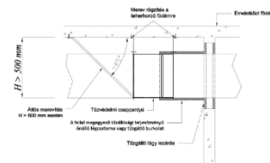
3D5.5.2. ábra Nagyméretű csappantyú beépítése merev rögzítéssel tűzszakaszhatáron kívül
