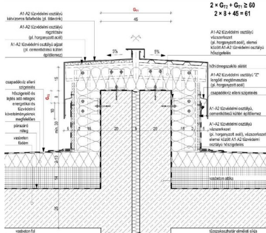
3F4 sz. ábra: lapostető tetősíkból kiemelkedő tetőszinti tűzterjedés elleni gátjának példája dilatációs egység határon
