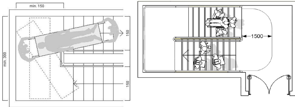
5A. ábra: Kerekesszékkal és hordággal történő mentésre alkalmas lépcsőház minimális méretei
