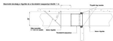
D5.3.1. ábra. Tűzcsappantyú és mereven rögzített acél légszatórna kapcsolódása rugalmas összekötő elemek nélkül
