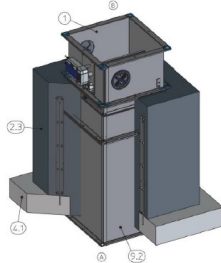
3D5.6.1. ábra. Tűzajtó csappantyú beépítése vasbeton gallerba a vasbeton fődém síkjától távol
