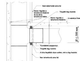
D5.3.4. ábra. Nem teherhordó álsíkfalba épített kis méretű tűzvédelmi csappantyú a födémhez és az alsó teherhordó falához mereven rögzített légszatórnákkal
