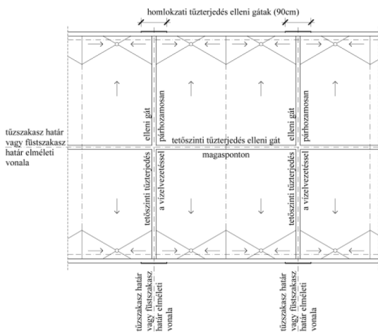
F9 sz. ábra: lapostetők vízelvezetése és a tűzterjedés elleni gátok összefüggései
