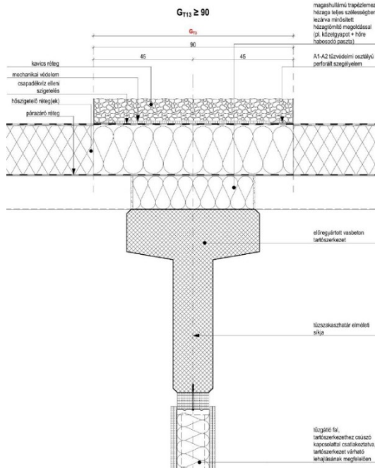
3F8 sz. ábra: előregyártott vasbeton vázszerkezetű és könnyű tetőfödém térelhatároló szerkezetű épület tűzszakaszhatárhoz kapcsolódó síkban tartott tetőszinti tűzterjedés elleni gátjának példája
