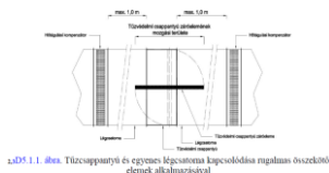
2D5.1.1. ábra. Tűzcappantyú és egyenes légszatórna kapcsolódású rugalmas összekötő elemek alkalmazásával
