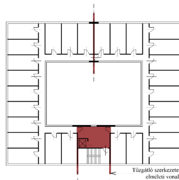
F2.3. ábra Épület szintenként két átmeneti védett tér és lépcsőház együttesével, de tűzszakaszolás nélkül
