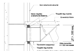
D5.3.3. ábra. Nem teherhordó álsíkfalba épített, a födémhez mereven rögzített nagy méretű tűzvédelmi csappantyú
