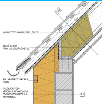
E2 sz. ábra. Falazott, éghető hőszigeteléssel ellátott fal és átszellőztetett légréses magastető csatlakozása
