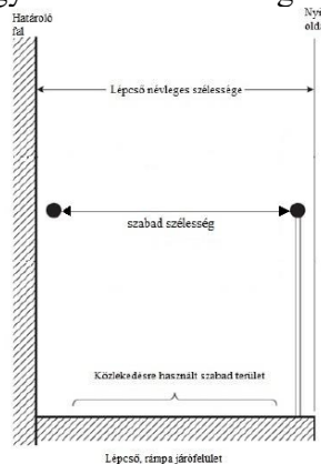
C6. ábra: Lépcsők, rámpák szabad szélessége
