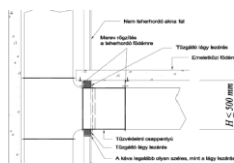
D5.3.2. ábra. Nem teherhordó álsíkfalba épített, a födémhez mereven rögzített kis méretű tűzvédelmi csappantyú
