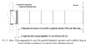
2D5.1.3. ábra. Tűzcappantyú és egy fű ponttal beépített egyenes acél szellőző légszatórna kapcsolódású rugalmas összekötő elem alkalmazásával
