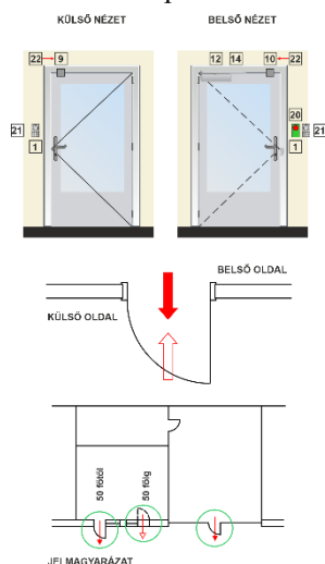
G18. ábra: Egyszárnyú, elektromos zárassal rendelkező homlokzati ajtók / tűzgátló ajtók – „B” típus
