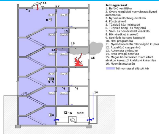
H-2. ábra: Példa előteres túlnyomásos füstmentes lépcsőház kialakítására, szabályozott üzemi ventilátorral, túlnyomás levezető kupolával
