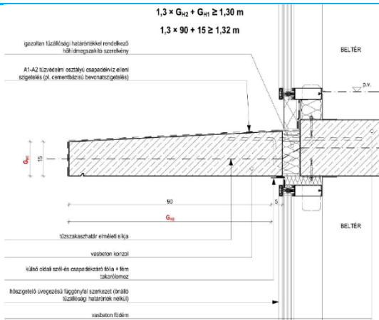
3F10 sz. ábra: üvegfal vonalában tartott hőhídmegezártítóval ellátott, megfelelő tűzállósági teljesítményű homlokzati tűzterjedés elleni gát példája
