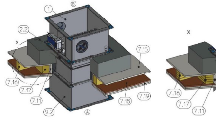
3D5.6.2. ábra. Tűzajtó csappantyú beépítése vasbeton gallerba egy fagerendás fődém síkjára
