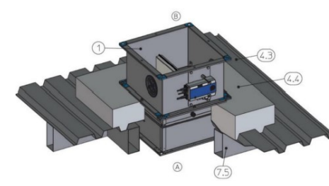
3D5.6.4. ábra. Tűzajtó csappantyú beépítése vasbeton gallerba könnyűszerkezetes fődém síkjára
