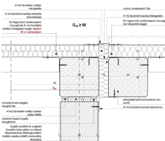
3F12 sz. ábra: előregyártott vasbeton pillérvázás tartószerkezethez kőzetgyapot maghőszigetelésű szendvicspanelből kialakított homlokzati tűzterjedés elleni gát példája
