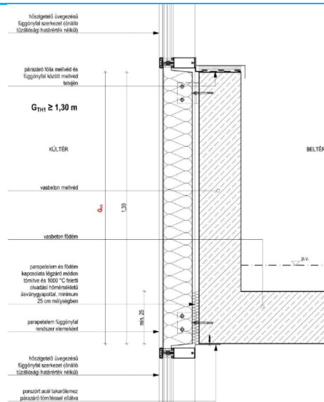
3F11 sz. ábra: tűzállósági teljesítmény nélküli függönyfaltól független, a tűzgátló födémmel folytonos egységet alkotó, önálló tűzállósági teljesítményű parapetfal, mint homlokzati tűzterjedés elleni gát példája
