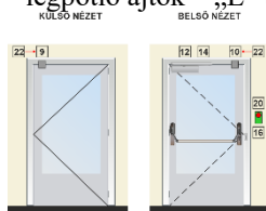
G21. ábra: Egyszárnyú, elektromos zárással rendelkező homlokzati ajtók / tűzgátó vagy légpótló ajtók – „E” típus
