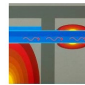
D1.5.1.2. ábra tűzterjedés hővezetéssel és hőszugárzással
