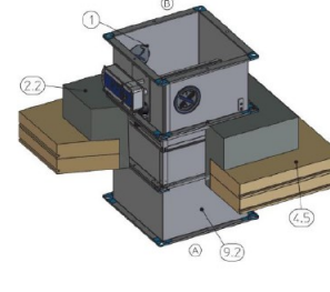
3D5.6.3. ábra. Tűzajtó csappantyú beépítése vasbeton gallerba CLT fődém síkjára
